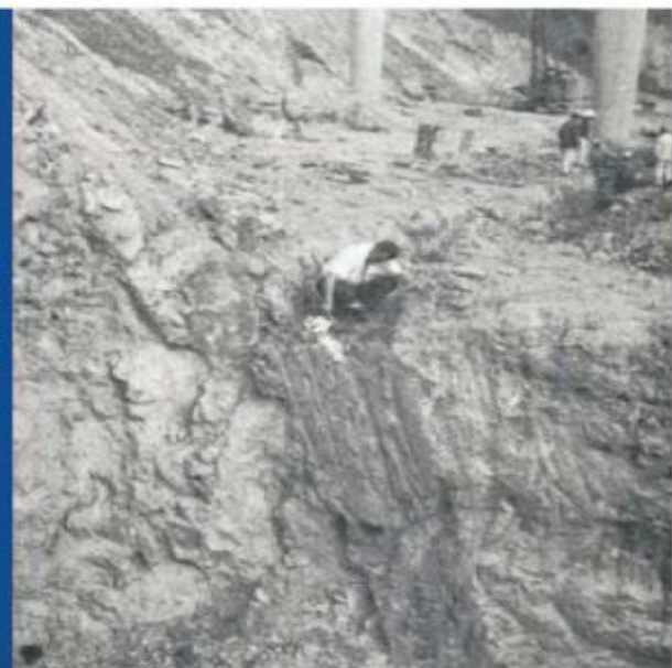
Vista al este de una brecha de falla arcillosa (gouge de falla) con buzamiento sur encontrada durante la construcción de la Av. Boyacá (Cota Mil) sobre la traza activa de la falla del Ávila en la salida hacia San Bernardino. Fuente: Circular N° 37 de la Sociedad venezolana de Geólogos (1969).
