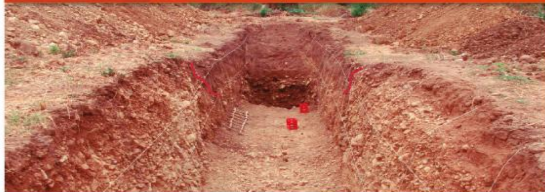
Vista longitudinal de la trinchera a través de la ruptura del sismo de Cariaco (ver foto anterior), estando la falla en el salto de la topografía (indicado por flechas) y en el cambio de material grueso a fino. Fuente: Franck A. Audemard (1997).
