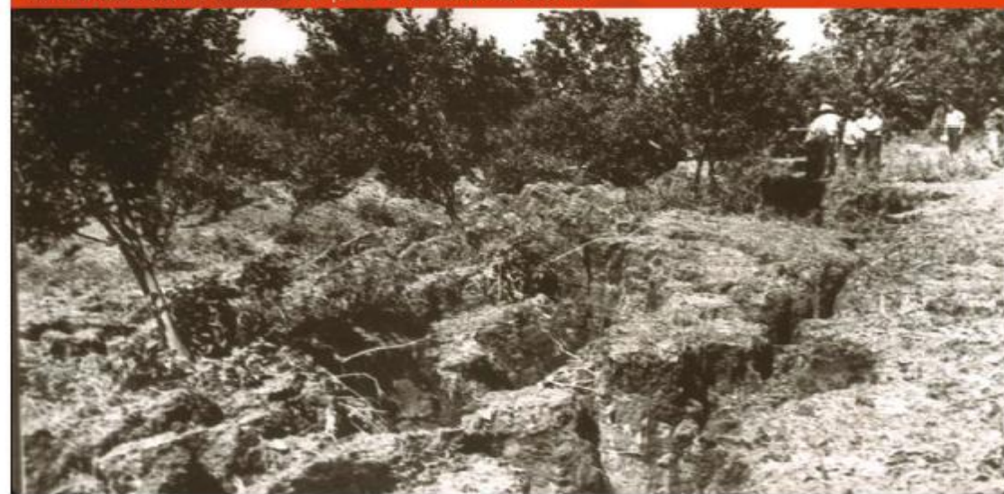
Detalle de la corona parte alta del relajamiento lateral de la costa sur del lago de Valencia, a consecuencia del terremoto de Caracas de 1967. Fotografía tomada de Hanson y Degenkolb en: Tomos Comisión Presidencial para el estudio del sismo.
